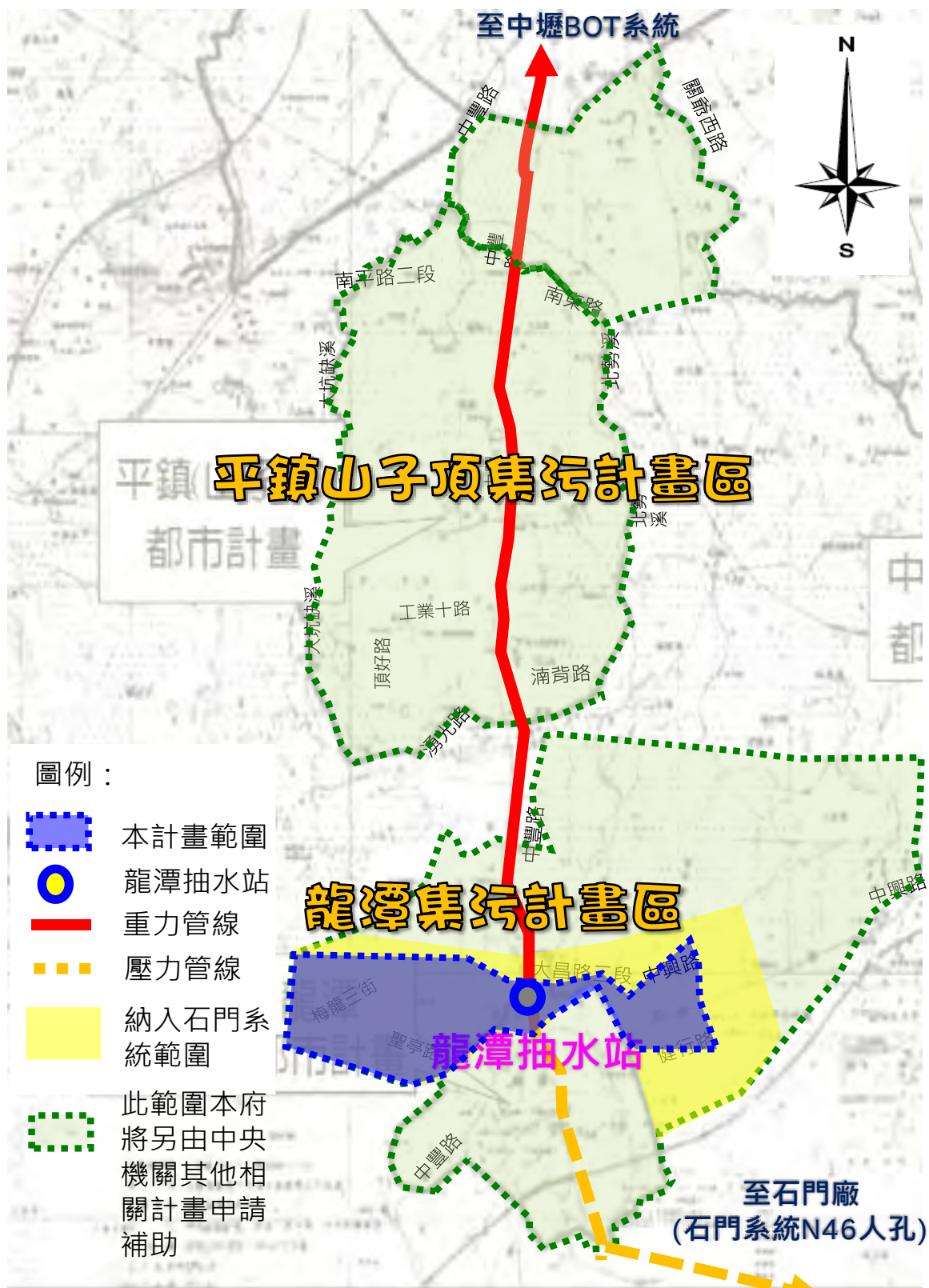
圖 16、龍潭污水下水道系統新建計畫規劃構想示意圖
