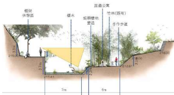
竹林親水步道斷面圖
